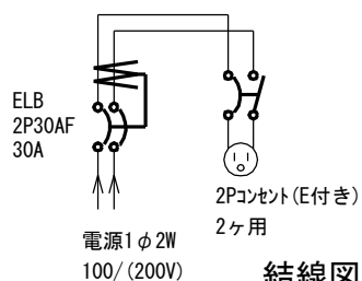
結線図
